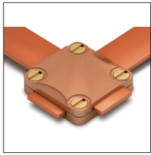
AT-034F Manguito cuadrado bronce pletina 25x6mm
