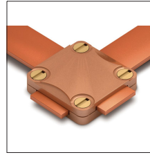
AT-033F Manguito cuadrado bronce pletina 25 x 3mm
