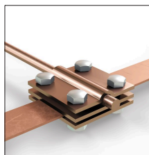
AT-133F Manguito cuadrado Cu, cable o pletina
