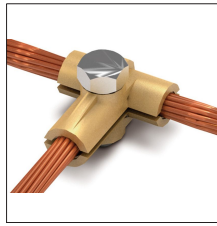
AT-012F Manguito en T de latón para cable ø8-10mm
