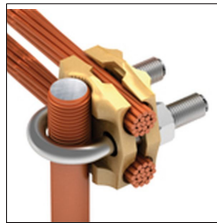
AT-092J Manguito latón tipo CGUV pca/cb 150- 300mm 2
